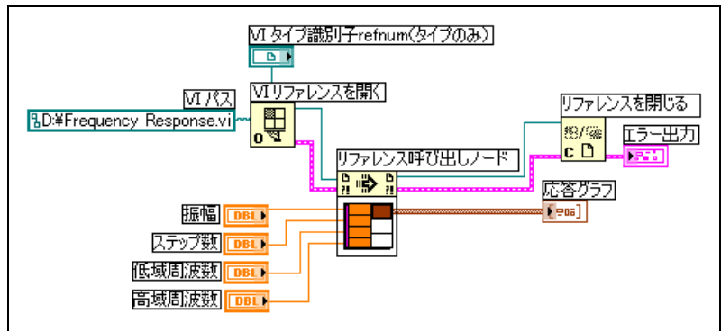
図 17-5 「リファレンス呼び出しノード」を使用する
