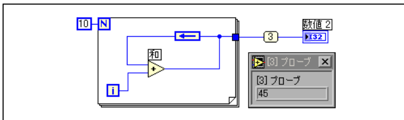
図 8-5 For ループで最後の値を渡す
