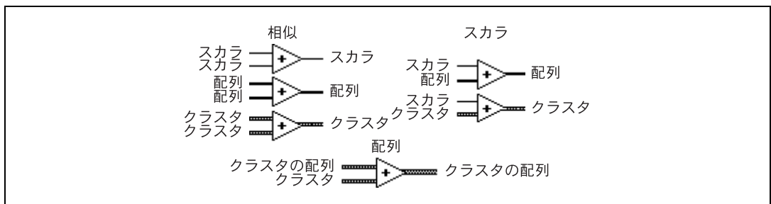
図 B-1 「和」関数での多形の組み合わせ
