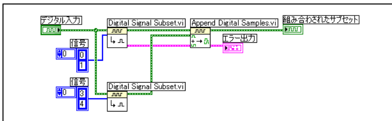
図 4-4 デジタル波形を連結する
