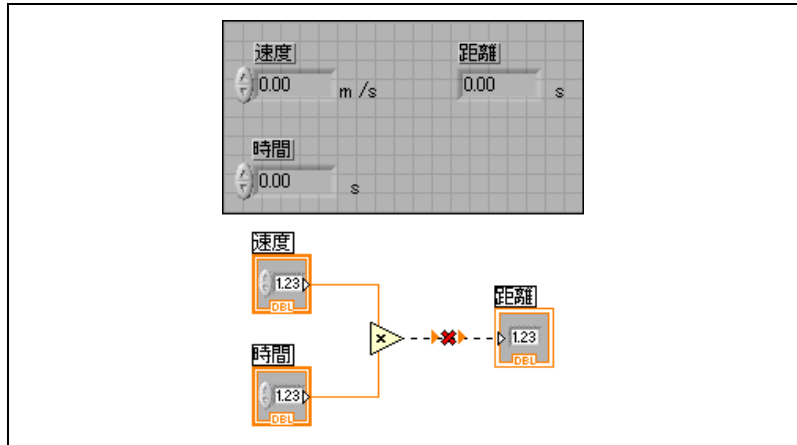
図 5-6 単位に互換性がないオブジェクトの配線による不良ワイヤ
